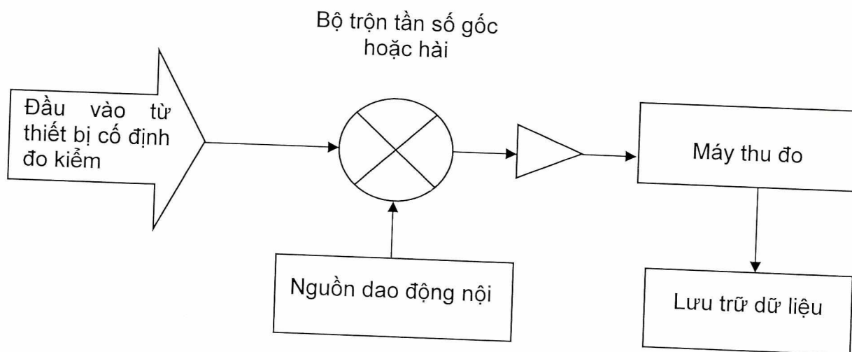
Hình 2 - Sơ đồ thiết lập đo kiểm của bức xạ ngoài băng và phát xạ giả
