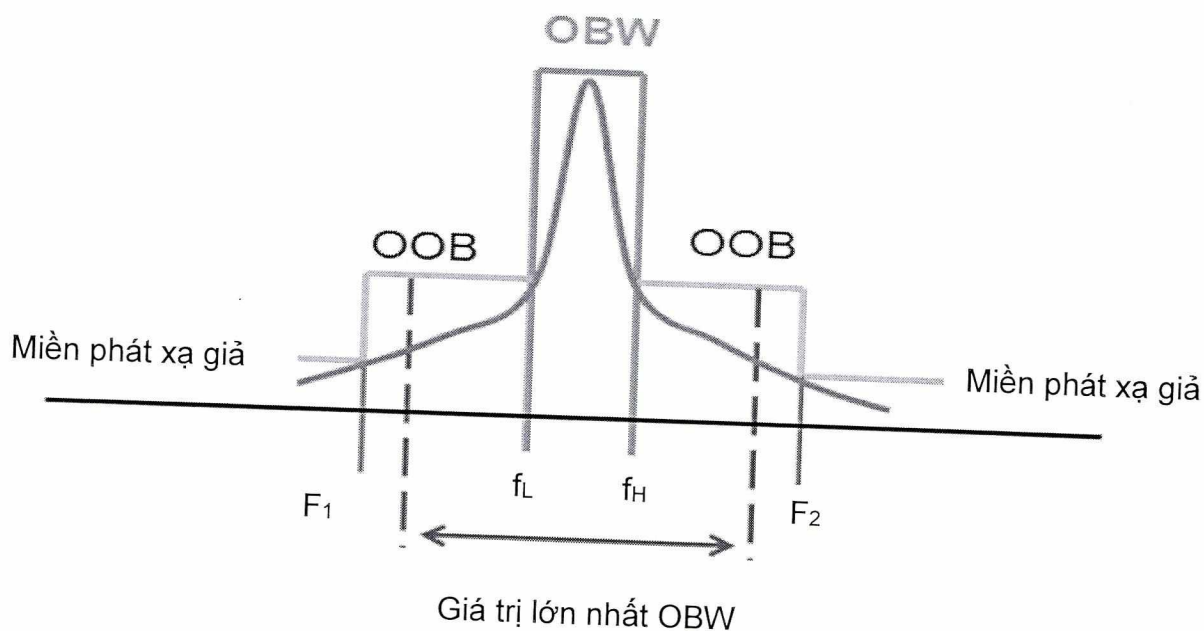
Hình 1 - Tổng quan sự phụ thuộc OOB/phát xạ giả vào OBW
