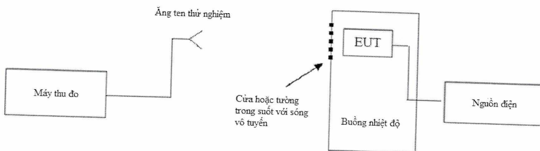
Hình C.3 - Thiết lập điều kiện đo kiểm khắc nghiệt
