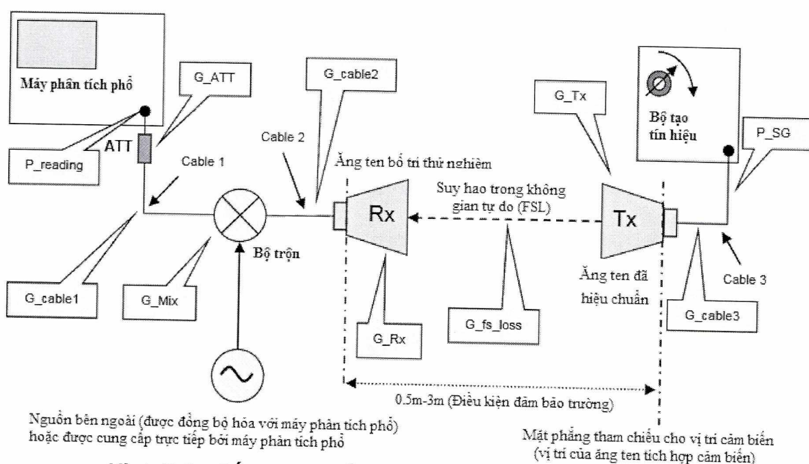
Hình E.2 - Cấu hình thiết lập hiệu chuẩn bao gồm bộ trộn
