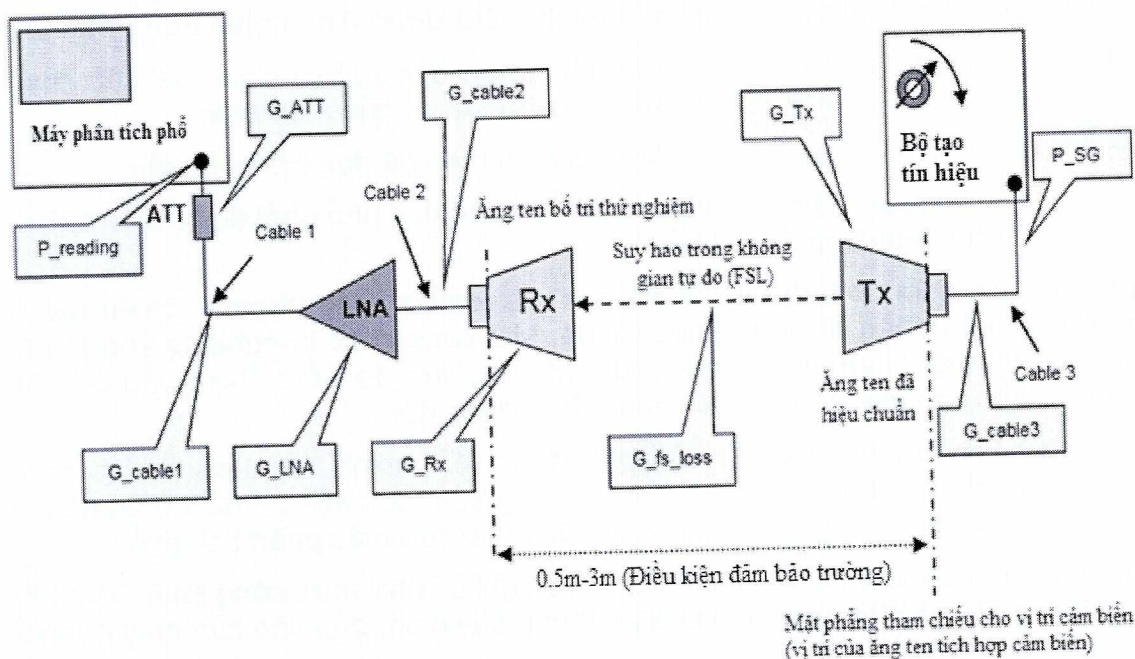
Hình E.1 - Cấu hình thiết lập hiệu chuẩn
